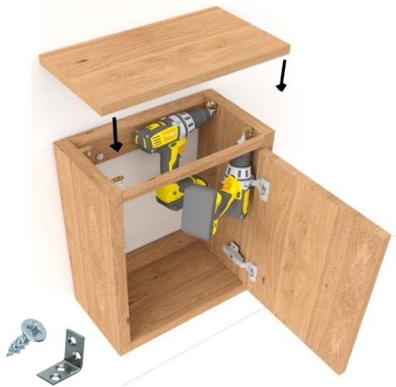
5. Eikenblad bevestigen aan meubel * montageset meegeleverd
