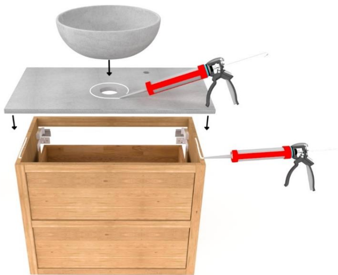
3. Blad en opzetkom met kit bevestigen op het meubel
