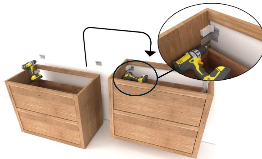
2. Montageplaten aan muur bevestigen en meubel ophangen*
